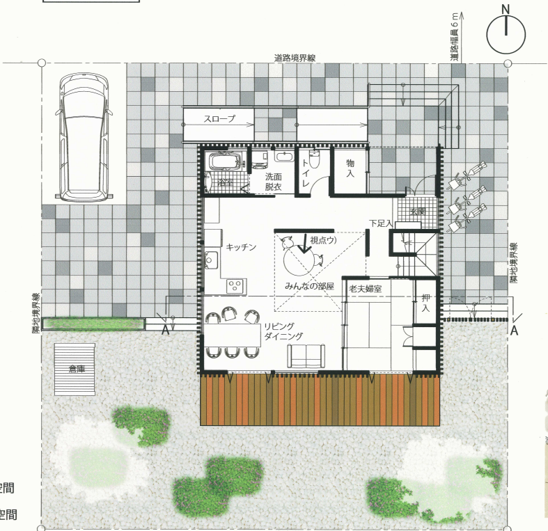
配置図兼 1階平面図 S=1/100
