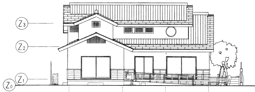
南立面図 1:100
