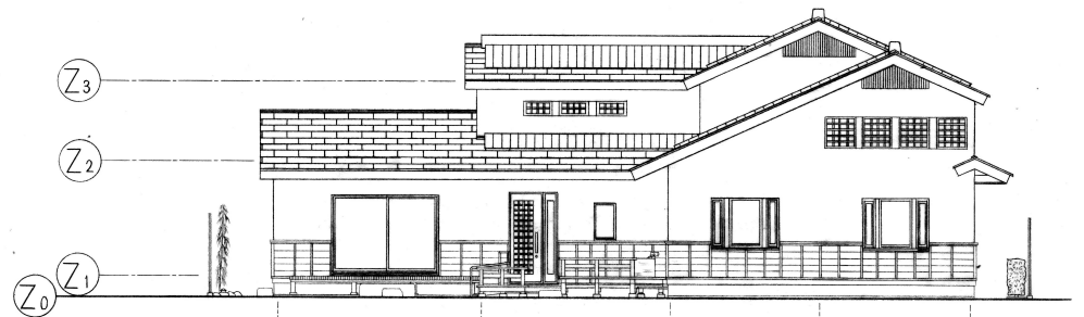
東立面図 1:100
