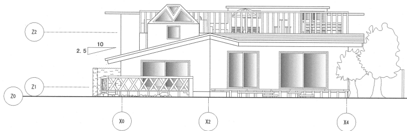
南立面図 (S=1:100)
