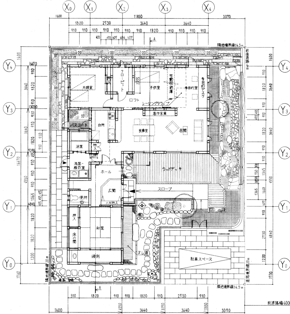
配置図兼平面図 1:100
