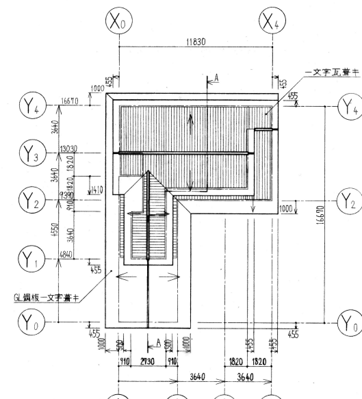
屋根伏図 1:200
