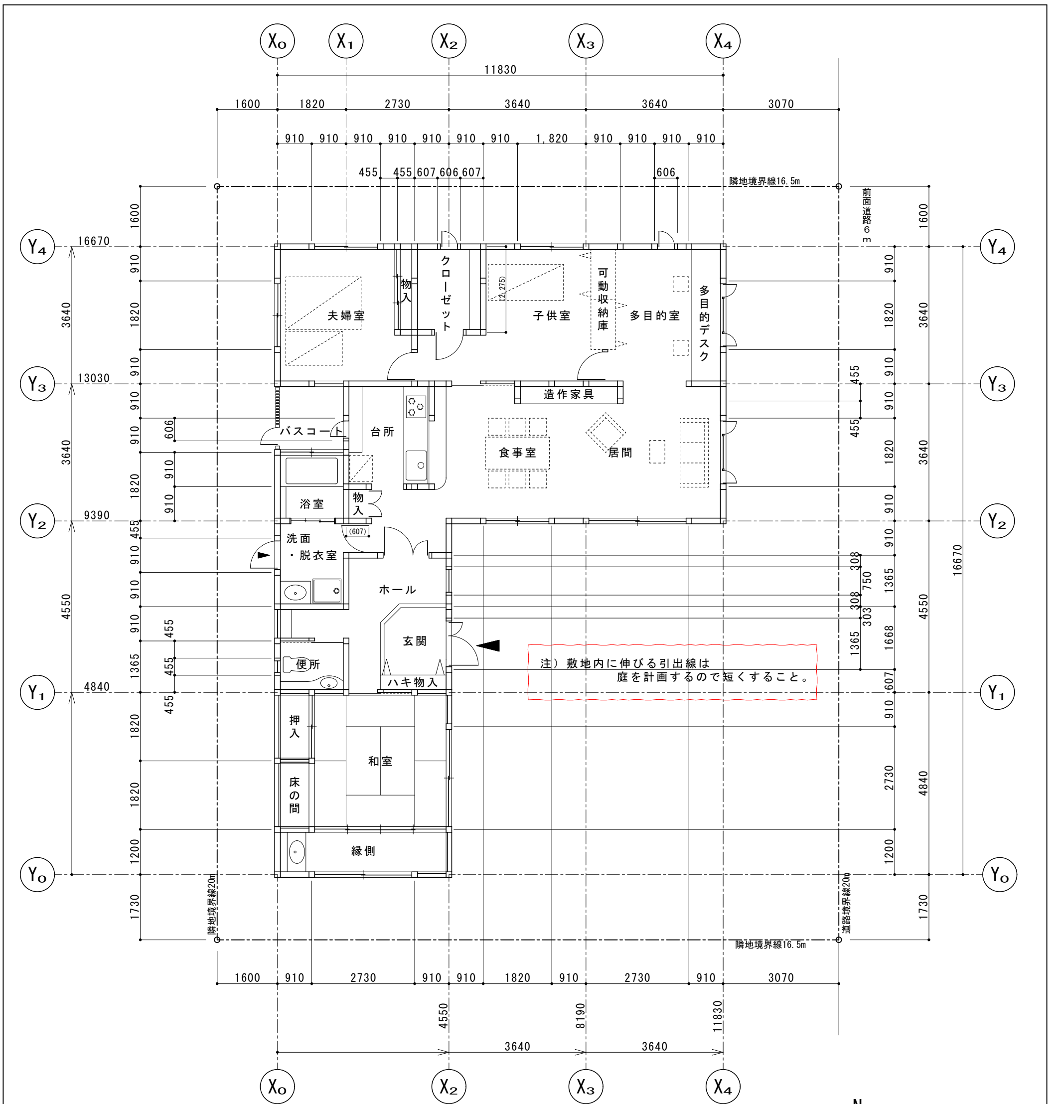
配置図兼平面図 S=1:100
