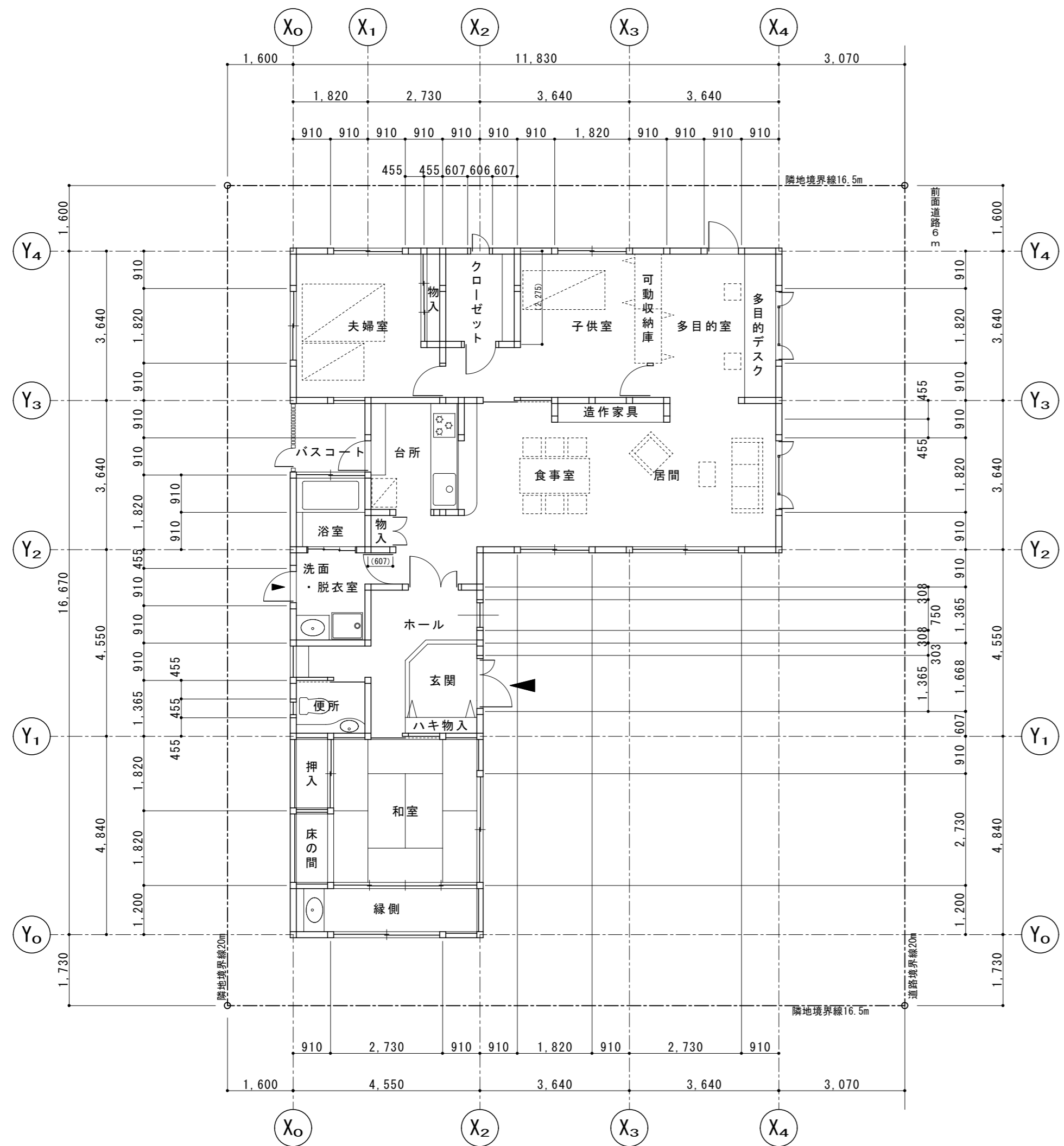
配置図兼平面図 S=1:100
